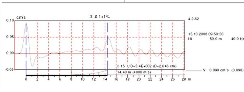
Wellenausbreitung bei der Integritätsprüfung nach dem „Low-Strain“-Verfahren
