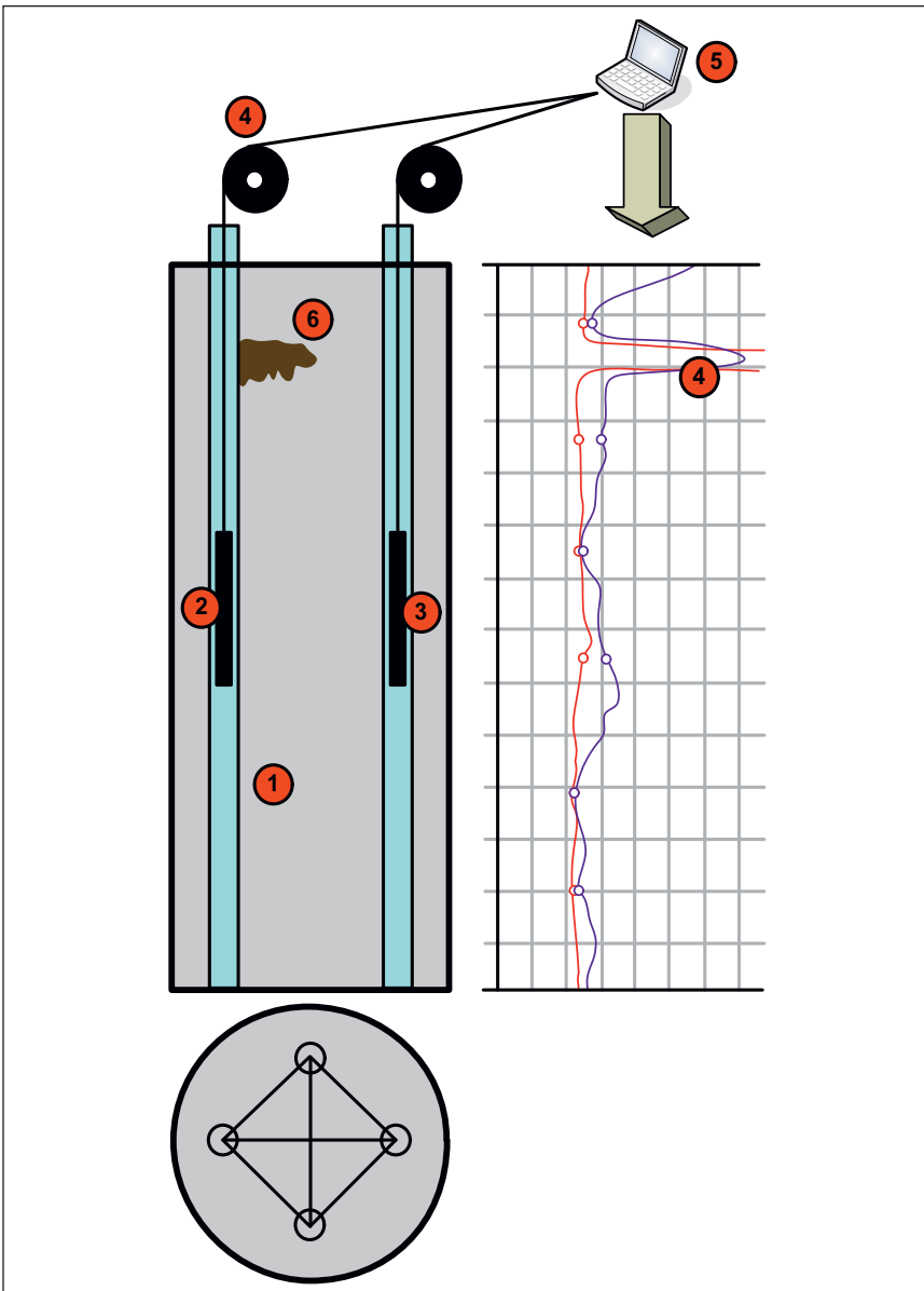
Schematische Darstellung einer Cross Hole Ultrasonic Messung (Quelle: www.piletest.com )
